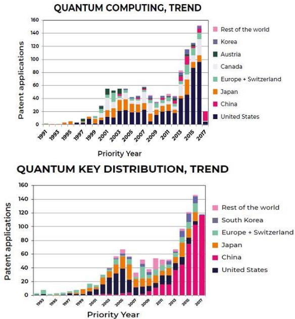
Figura 1: Numero di brevetti rispettivamente in ambito quantum computing e quantum key distribution, per Paese fino al 2017. Si osserva un lento abbandono della quantum key distribution (QKD) da parte degli Stati Uniti, che si sono concentrati sui computer quantistici, mentre la Cina ha invece investito principalmente proprio in tali comunicazioni quantistiche. Recentemente la Cina ha reimpiegato le tecnologie per la QKD anche per i computer quantistici. Il Giappone ha prodotto più brevetti dell'intera Europa. Fonte: Roadmap della Commissione Europea sulle Tecnologie Quantistiche (2018).
